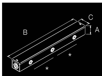
DUCTO PARA 3 MEDIDORES
