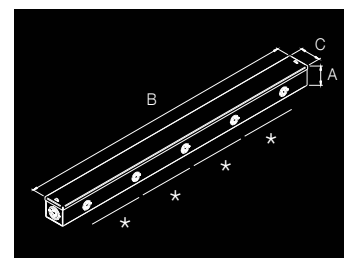
DUCTO PARA 5 MEDIDORES
